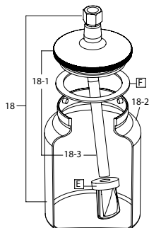
Saugbecher 1 lt. mit Bajonett Schließung (Für Saug-Modelle)
