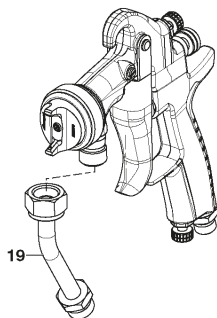
Farbrohr (Fakultativ für Druck-Modelle)
