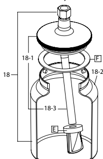
AG-1 - Reservoir à succion de 1 litre (pour les modèles à succion)
