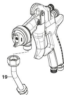
Tubería fluido (opcional para los modelos a presión)
