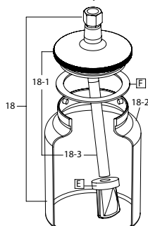
AG-1 - Depósito de 1lt con cierre a Bayoneta (Para los modelos a succión)
