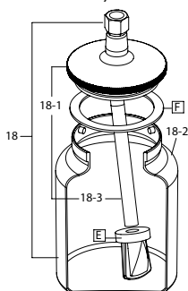
AG-1 - Copo de sifão com fecho baioneta (para os modelos de sifão)
