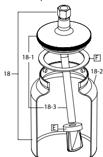
AG-1 - Tazza da 1lt con chiusura a Baionetta (per modelli a sifone)
