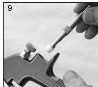
9. Installer le nouveau joint avant sur l'outil d'entretien de façon à ce que la rainure soit orientée vers la poignée de l'outil.
