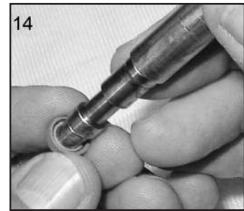
14. Instale una junta trasera nueva en la herramienta de mantenimiento de manera que la muesca quede orientada hacia el extremo con mango de la herramienta.
