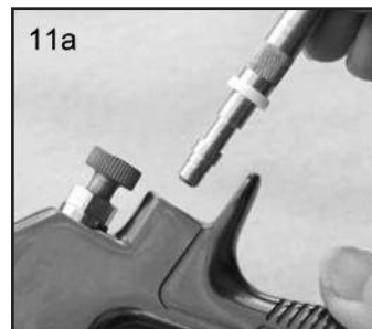
11a. Installer le nouveau siège de soupape sur le corps de la soupape.
