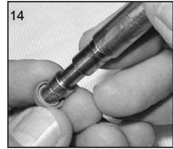
14. Installer le nouveau joint arrière sur l'outil d'entretien de façon à ce que la rainure soit orientée vers la poignée de l'outil.
