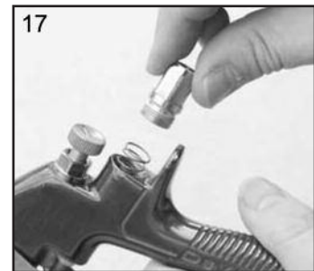
17. Vuelva a colocar el muelle de la válvula insertando el extremo pequeño del muelle en la pistola, y el tornillo en el alojamiento (10).
