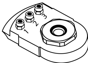
3. Konfigurace nářadí pro použití ochranné přechodky nebo vložky, šrouby a matice namontovány v poloze 1, 2, 3.
